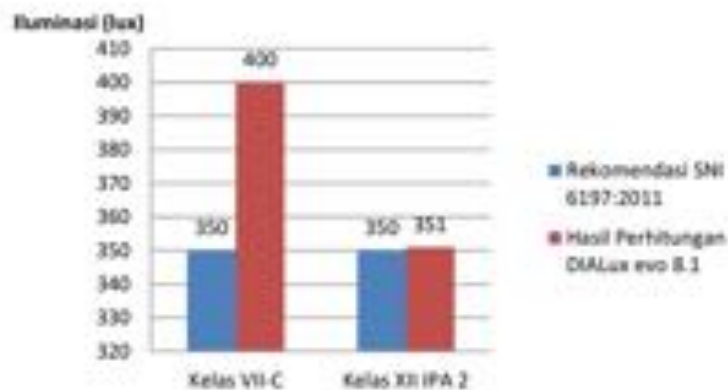
Gambar 11 Grafik Perbandingan Hasil Perhitungan terhadap minimal rekomendasi SNI 6197:2011
