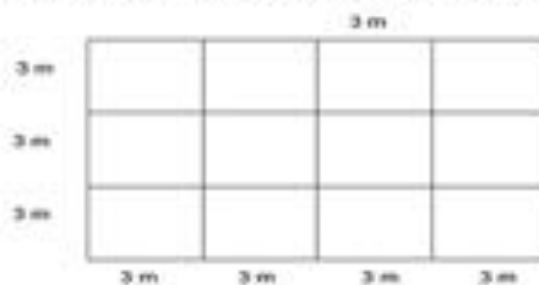
Gambar 3 Penentuan titik pengukuran dengan luas antara 10 \text{ m}^2 hingga 100 \text{ m}^2
